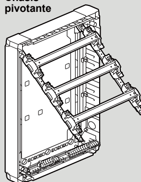
Chasis pivotante
