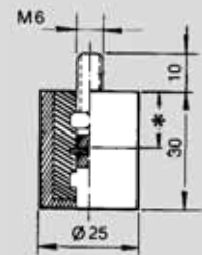
SBC-2 Tuerca M6 Tornillo M6x15
