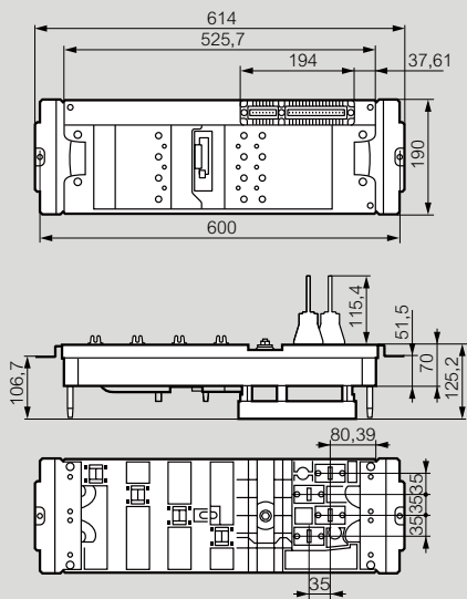
Bases para DPX 3 160
