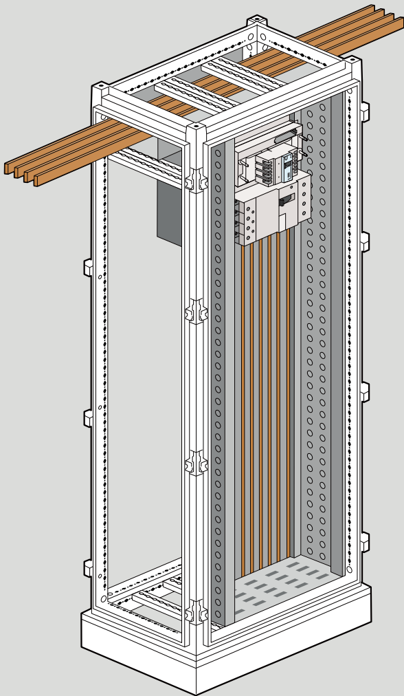
Bases para DPX 3 160
