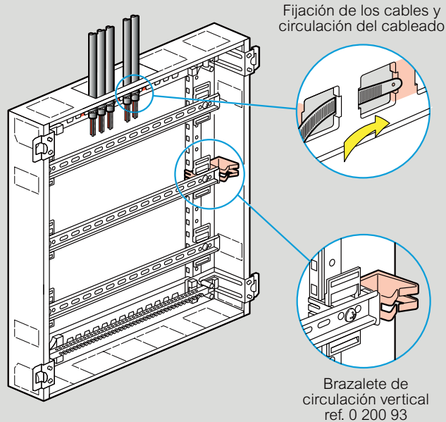
Chasis extraíble
