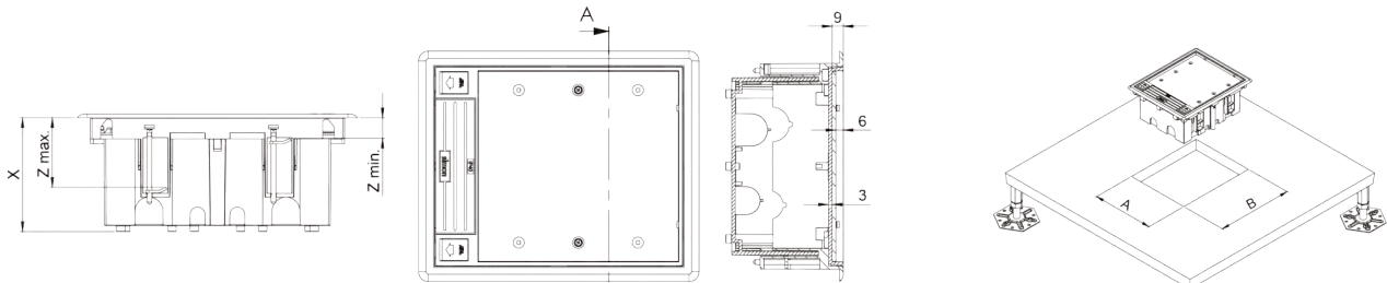
Cajas de 90 mm / 120 mm (Piso falso)
