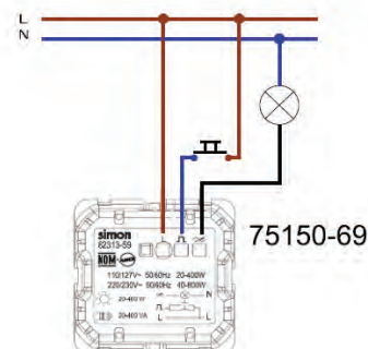
Función Pulsador 3 Vías Para control desde dos puntos con un dimmer y un pulsador auxiliar
