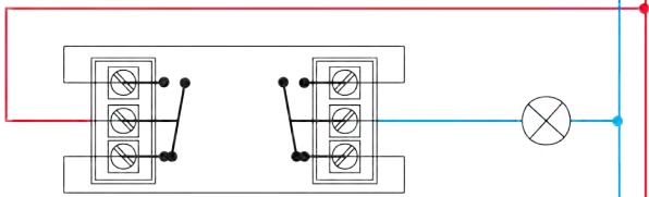
Interruptor 3 vías con luz piloto
