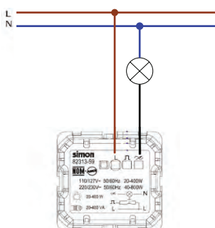
Función Pulsador 2 Vías Para controlar con un solo dimmer
