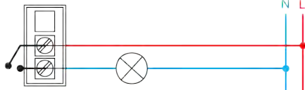
Interruptor 2 vías con luz piloto
