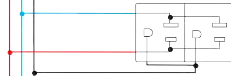
Toma de corriente dúplex 2p+tierra
