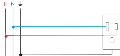
Toma de corriente 2p+tierra
