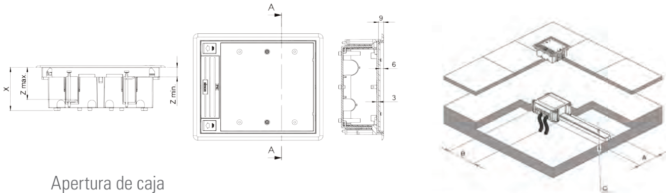
Cajas de 70 mm / 100 mm (Pavimento)
