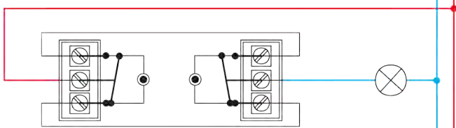
Interruptor 3 vías con luz piloto
